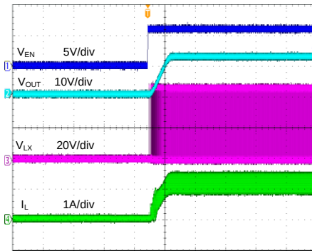
Startup from EN ( V_{IN}=48V , V_{OUT}=12V , I_O=1.2A )
