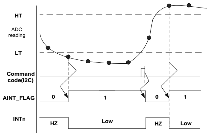
Figure 4. ALS Window Interrupt
