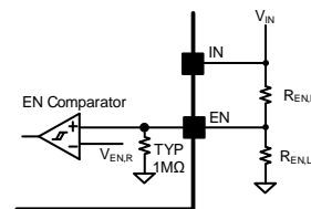
Figure4. Enable Control
