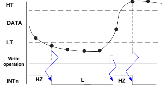
Figure. 5 ALS Interrupt Example
